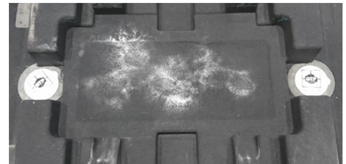
NETCore® Brechkern nach dem Einformen
